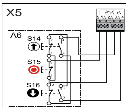
Trojtlačítko zablokováno
