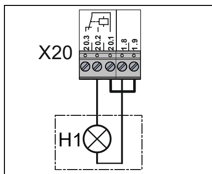
Signální světlo
