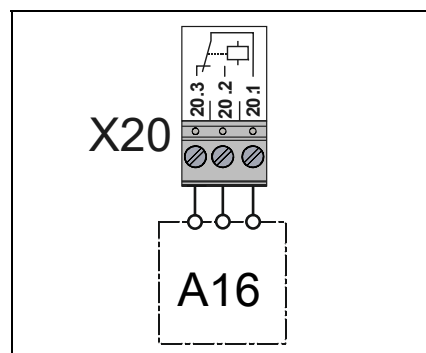
Externí přístroje
